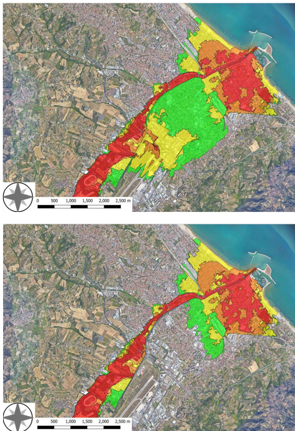
Figura 5-9: Fasce di pericolosità. In alto sono riportati i risultati ottenuti in configurazione attuale, in basso quelli in configurazione futura (considerando gli effetti delle vasche di Cepagatti, della chiusura dei sottopassaggi in corrispondenza dell'area aeroportuale, delle opere previste dal PRP del porto di Pescara).
