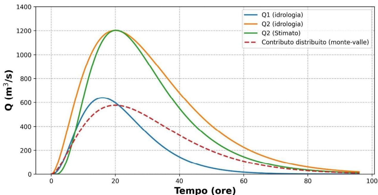
Figura 3-2: Risultato del secondo passo di applicazione del metodo di stima del contributo distribuito.
