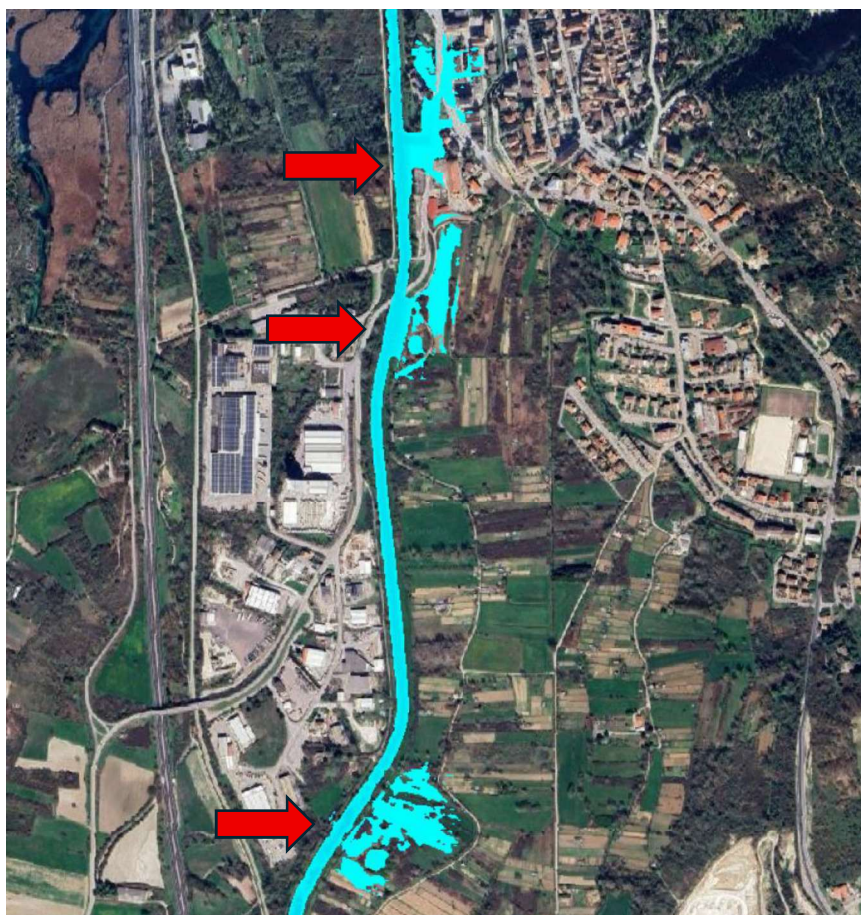
Figura 5-11: Identificazione di punti in cui ha origine il processo di esondazione nei pressi del comune di Popoli.
