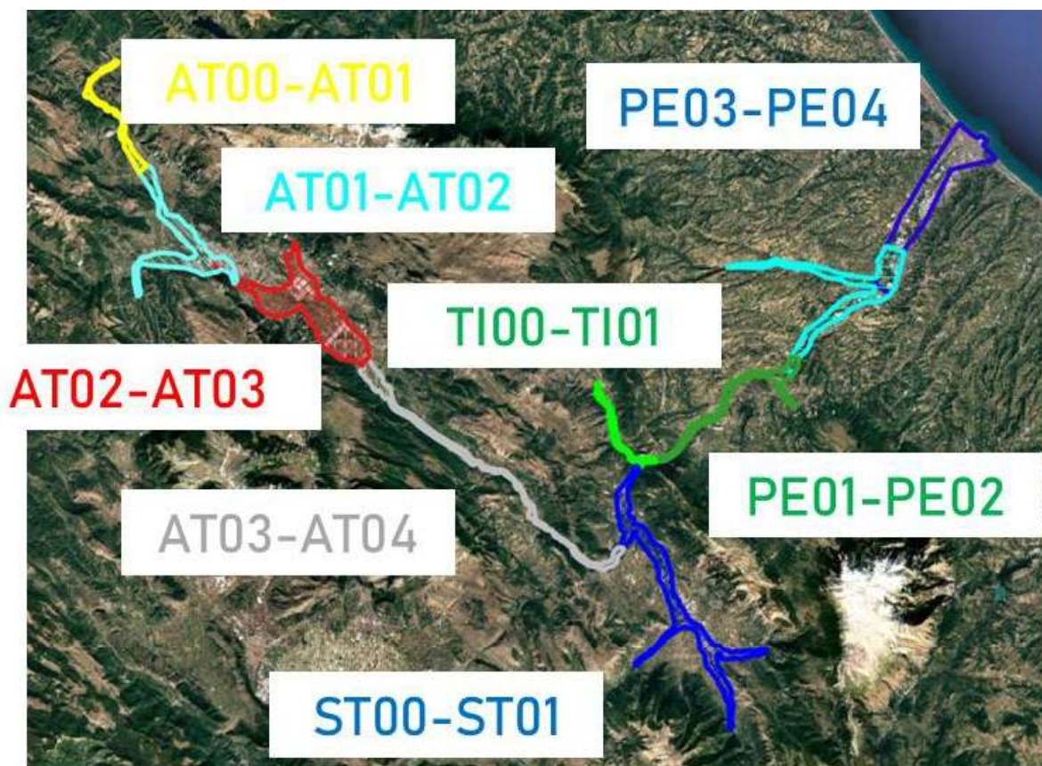
Figura 4-4: Domini di calcolo implementati.
